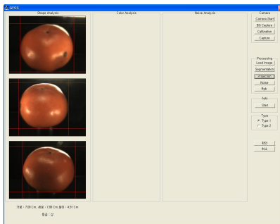
그림 8. 과일 크기 분석 Fig 8. Analysis of Size of Fruit
