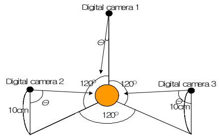
그림 1. 부피 측정을 위한 카메라들의 배치 Fig 1. Arrangement of Camera for Calculating the Volume
