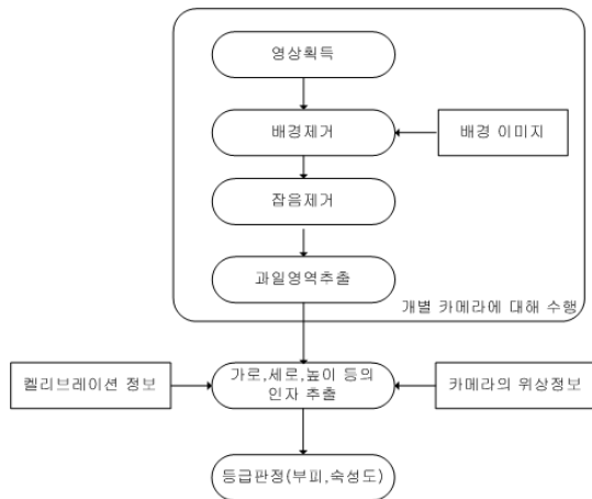
그림 3. 선과시스템 알고리즘 Fig 3. Algorithm of a Fruit Classification System
