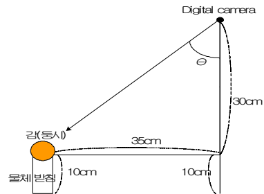
그림 2. 카메라와 과일의 배치 Fig 2. Arrangement of the Cameras and a Fruit
