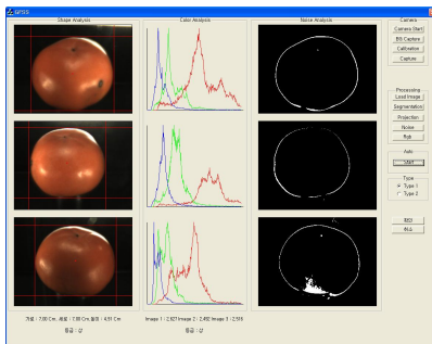
그림 9. 크기, 숙성도의 등급 판정 결과 화면 Fig.9 Result Screen of Decision Grade about Size and Maturity
