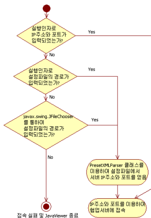
그림 12. 확장된 JavaViewer의 접속절차 Fig. 12. Connection process of the extended JavaViewer
