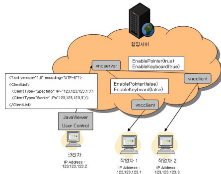
그림 8. 권한 변경 시나리오 Fig. 8. Access authority modification scenario
