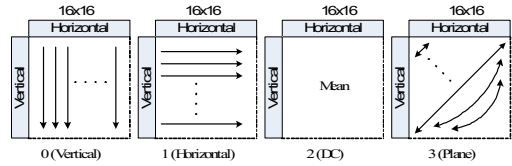
그림 4. 인트라 16x16 예측 부호화 Fig. 4. Intra 16x16 Prediction
