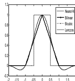
그림 1. 가중치 함수 \kappa(r) Fig. 1. Weight Function \kappa(r)
