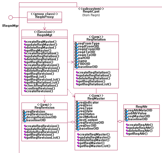
그림 13. 무기체계 연구개발 형상/정보관리시스템 컴포넌트 내부 클래스 다이어그램 일례
