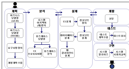
그림 7. 무기체계 연구개발 형상/정보관리시스템 개발프로세스 아키텍처
