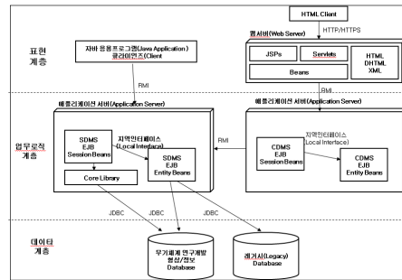
그림 5. 무기체계 연구개발 형상/정보관리시스템 실행시점 아키텍처 Fig. 5. Run-time Architecture of R&D Information System
