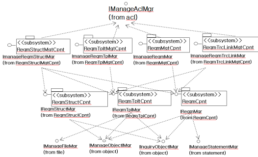
그림 11. 무기체계 연구개발 형상/정보관리시스템 컴포넌트 아키텍처 다이어그램 일례 Fig. 11. Component Architecture Diagram of R&D Information System
