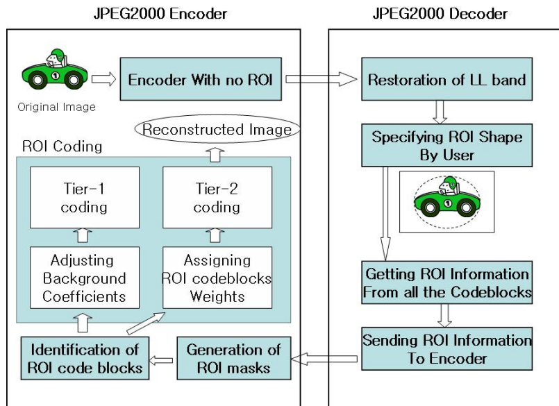
그림 2 제안된 기법이 포함된 JPEG2000 구성 Fig. 2 JPEG2000 construction with proposed method
