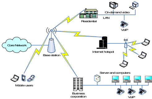
그림 1. 이동 WiMAX 환경 Fig 1. Mobile WiMAX Environment
