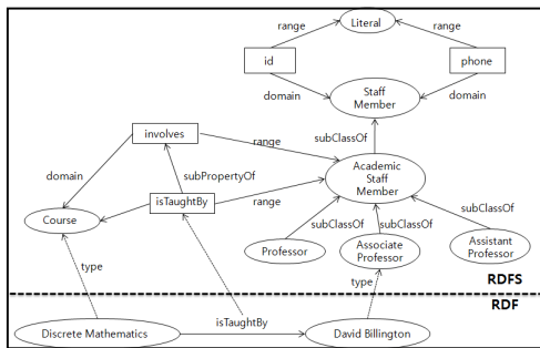
그림 1. RDF 레이어와 RDFS 레이어 Figure 1. An example RDF model consisting of RDF layer and RDFS layer
