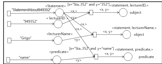
그림 7. reification의 컬러 페트리 넷 모델 Figure 7. A CPN model for 'reification'
