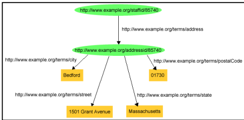
그림 5. RDF 문장의 객체가 구조체인 경우의 예 Figure 5. An example structured object in an RDF statement
