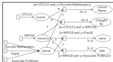
그림 4. rdf:Resource의 컬러 페트리 넷 표현 사례 Figure 4. An example CPN representation of rdf:Resource
