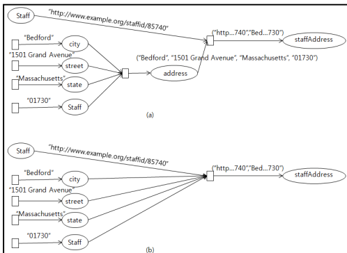
그림 6. 〈그림 5〉의 컬러 페트리 넷 모델. (a)주소가 다른 곳에서 참조될 경우 (b)그렇지 않은 경우 Figure 6. A CPN representation of the RDF statement shown in Figure 5, (a)adequate if 'address' is referred by some other statements, (b)adequate if 'address' is not referred by any other statements
