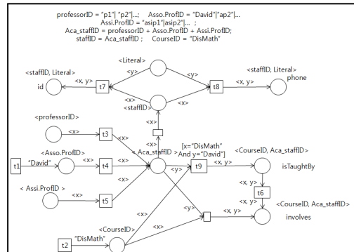
그림 3. 〈그림 1〉의 RDF 모델의 컬러 페트리 넷 표현 Figure 3. A CPN representing the RDF model in Figure 1
