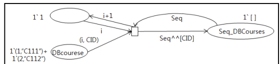
그림 2. rdf:Seq의 컬러 페트리 넷 모델 Figure 2. A colored Petri net model for rdf:Seq
