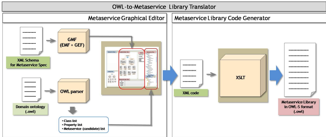
그림 5. OWL-to-메타서비스 라이브러리 변환 프로세스 Fig. 5. Translation Process of OWL-to-Met service Library
