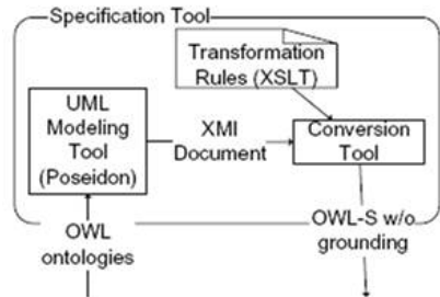
그림 2. UML to OWL-S 변환 과정 Fig. 2. Basic Architecture of the UML to OWL-S Conversion
