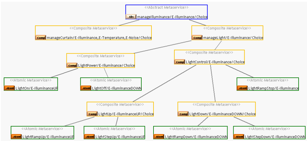
그림 11. 메타서비스 그래픽 요소로 편집한 메타서비스 샘플 (일부분) Fig. 11. Metaservice Sample using Metaservice Graphical Element
