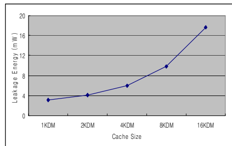
그림 1. 캐시 크기에 따른 정적 에너지 Fig.1 Static Energy Consumption of Various Cache Sizes
