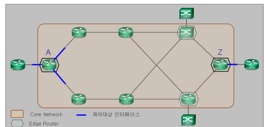
그림 10. 실험 네트워크 토폴로지 Fig 10. Network Topology of Testbed
