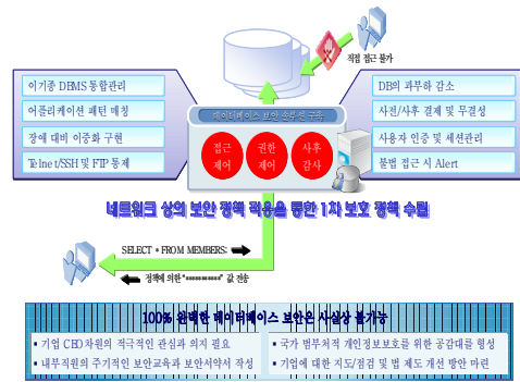
그림 5. 종합적인 DB 보안 프레임워크 Fig 5. Comprehensive DB security framework
