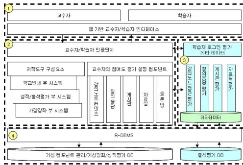
그림 3. 시스템 전체 구성도 Fig. 3. An Architecture of ProtoType Edumaker
