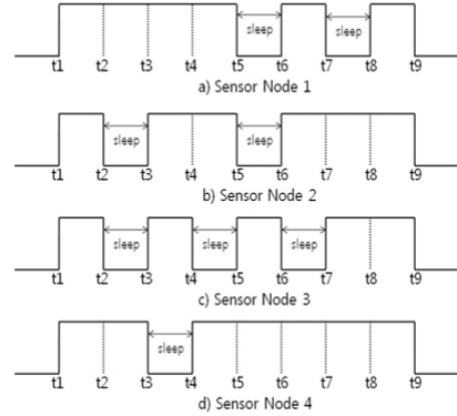
그림 5. 센서 노드의 Active/Sleep Fig. 5. An Example Active and Sleep Time of Sensor Node.
