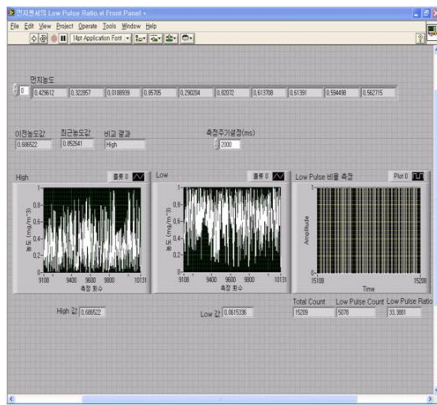
그림 6. LabVIEW 시뮬레이션 Front Panel Fig. 6. LabVIEW Front Panel.
