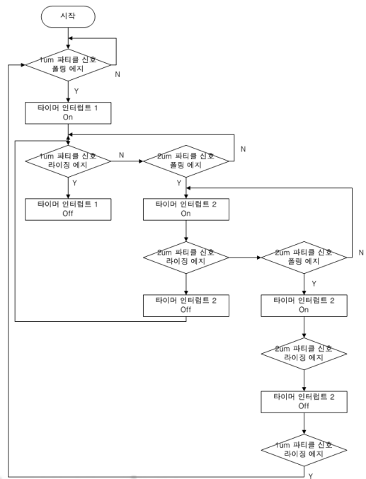
그림 3. 데이터 처리 알고리즘
