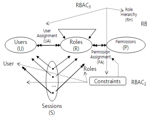
그림 1. 역할기반 접근통제 모델 Fig. 1. Role Based Access Control Model
