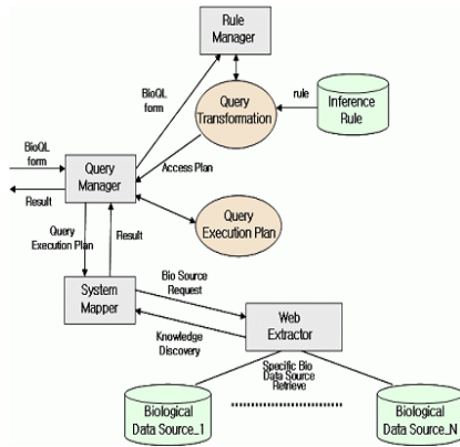
그림 7. 질의수행구조 Fig. 7. Query execution procedure
