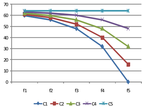
그림 2. 클래스 간에 동등한 간격으로 구성된 특징값 분포 예 Fig. 2. Examples of feature value distribution with equal inter-class intervals
