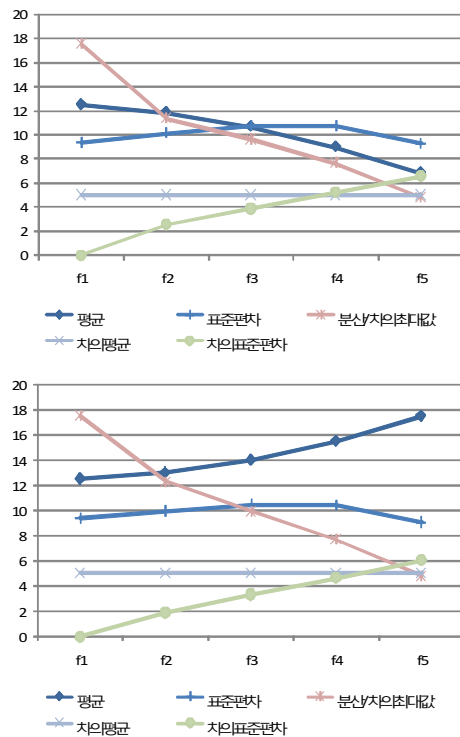
그림 5. 그림 3에 대한 5 가지 통계 정보 Fig. 5. 5 kinds of statistical information for Fig. 3
