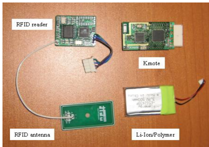
그림 2. 무선 센서 노드와 RFID 리더기 Fig. 2. Wireless sensor node and RFID reader.
