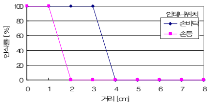
그림 7. RFID 태그와 리더 거리에 따른 인식률 Fig. 7. Recognition rate vs. distance between reader and tag.
