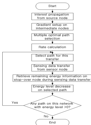
그림 2. 개선된 MP-DD 라우팅 알고리즘 절차
