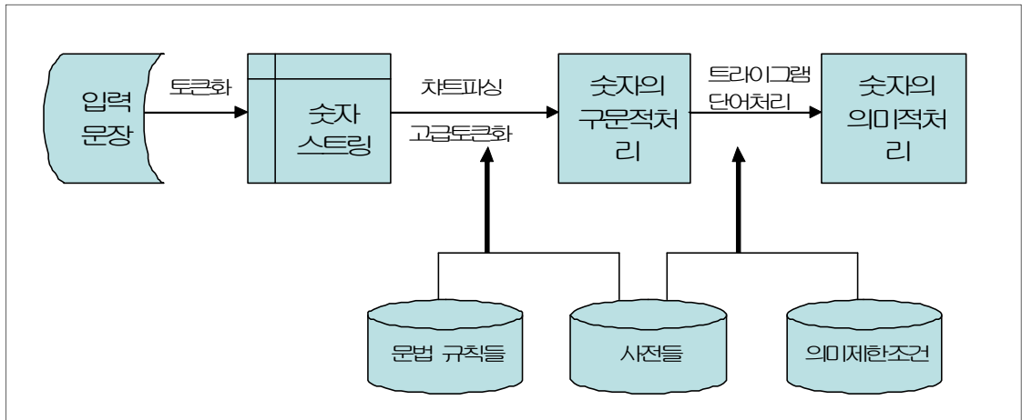
그림 1. 숫자 스트링 정보시스템 개요 Fig. 1. Outline of the Information System for Numeral Strings
