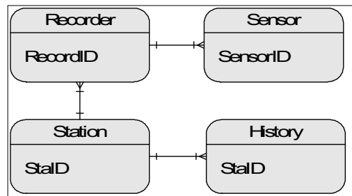
그림 6. 지진관측소 정보관리 개체-관계도 Fig 6. ERD for managing of seismic station
