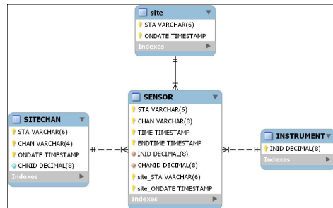
그림 5. CSS3.0의 주요 개체-관계도(ERD)(11) Fig 5. Entity-Relation-Diagram of CSS3.0(11)
