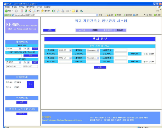
그림 14. 센서정보 입력 Fig 14. Registering of sensor information
