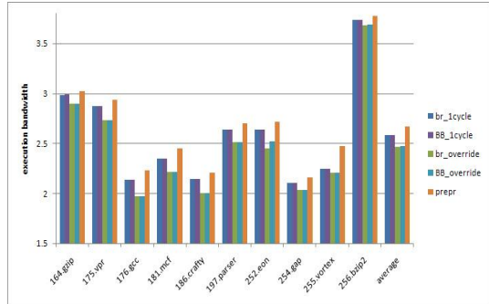
그림 6. 실행 대역폭 Fig. 6. Execution Bandwidth
