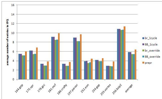
그림 5. 명령어 인출 대기열의 사용률 Fig. 5. Utilization of Instruction Fetch Queue
