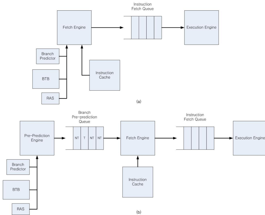
그림 1. 분기 선예측 시스템 Fig. 1. Branch Pre-Prediction
