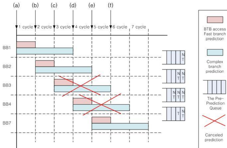
그림 3. 선예측 장치의 시간 도표 Fig. 3. Timing Diagram in Pre-Prediction Engine
