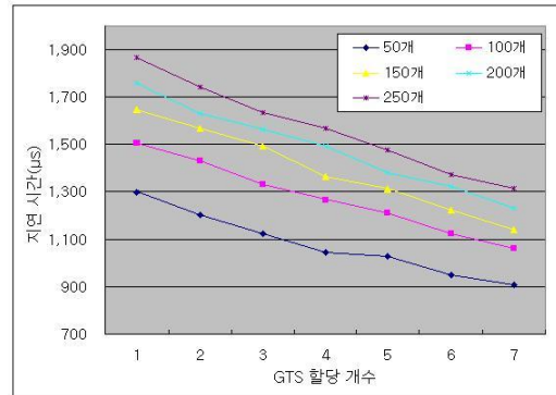
그림 4. GTS 개수와 PNC 선출 지연 시간 Fig 4. GTS number and PNC election delay time
