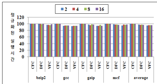
그림 9. 정규화 한 실행시간 (CINT) Figure 9. Normalized execution time (CINT)
