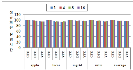
그림 10. 정규화 한 실행시간 (CFP) Figure 10. Normalized execution time (CFP)
