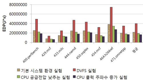
그림 6. 벤치마크 실험 시 Energy Delay Product(EDP) Fig. 6. Energy Delay Product(EDP) of each benchmark executions
