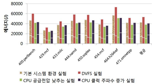
그림 5. 벤치마크 실행 시 에너지 (각각의 바에서 2등분 중 아래쪽은 CPU 에너지, 위쪽은 CPU 제외한 나머지 에너지) Fig. 5. Energy of each benchmark executions
