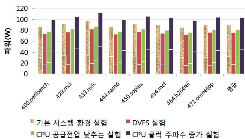
그림 4. 벤치마크 실행 시 평균 전력 (각각의 바에서 2등분 중 아래쪽은 CPU 전력, 위쪽은 CPU 제외한 나머지 전력) Fig. 4. Average power of each benchmark executions
