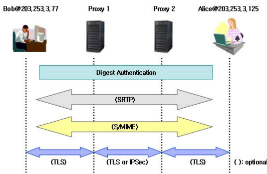
그림 5. SIP 보안 기술의 적용 영역 Fig. 5. An area effected by SIP security technologies
