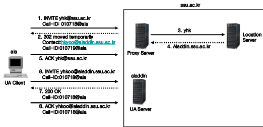
그림 4. 리다이렉트 모드에서 SIP 동작 Fig. 4. SIP operation on the redirect mode
