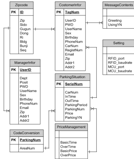
그림 8. ERD(Entity Relation Diagram) Fig. 8. ERD(Entity Relation Diagram)
