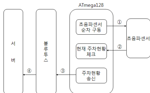
그림 9. 차량 진입이 없을 경우의 흐름도 Fig. 9. Diagram of the case of not enter a car
