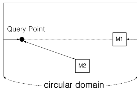
그림 1. 순환적인 검색공간 Fig. 1. Circular Search Space
