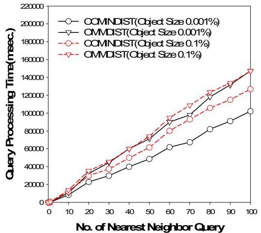
(b) 지수분포
