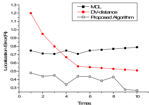
그림 10. 기존 알고리즘과 비교 Fig. 10. Comparison with existing algorithm.
