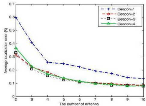
그림 8. 안테나 수에 따른 평균위치오차 Fig. 8. The average position error according to number of antenna.
