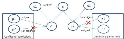
그림 4. 다른 역할에 다른 인가권한이 할당되는 문제 Fig. 4. Problem of assigning conflicting permissions to a same senior role
