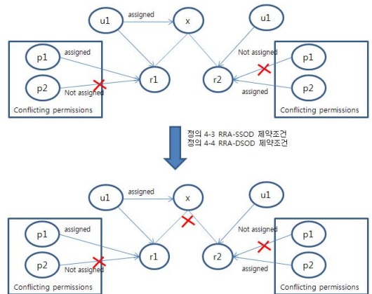
그림 10. 다른 역할에 각각의 인가권한이 할당되는 경우 동일 사용자 할당 문제 해결 Fig. 10. Resolution of assigning conflicting permissions to a same senior role
