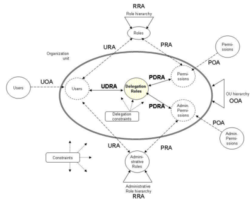
그림 6. OS-DRAM 모델 Fig. 6. OS-DRAM Model
