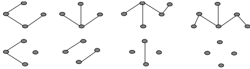
그림 7. OS-DRAM 모델에서 허용되는 역할계층 유형 Fig. 7. Types of role hierarchy of OS-DRAM model
