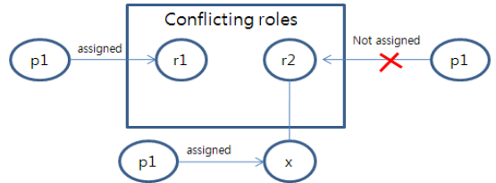
그림 3. 충돌 역할에 동일한 인가권한 할당되는 문제 Fig. 3. Problem of assigning a permission to conflicting roles
