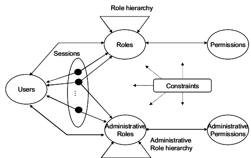
그림 1. ARBAC97 모델 Fig. 1. ARBAC97 Model
