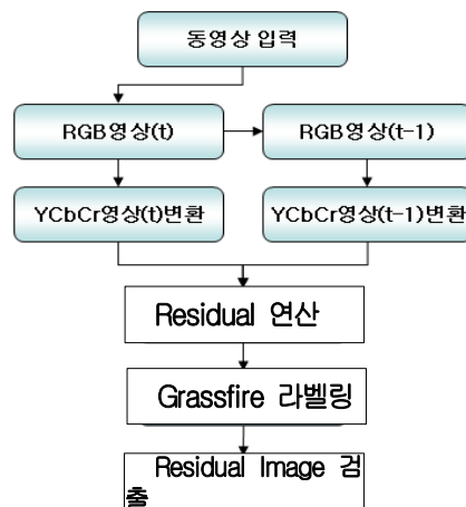
그림 2. Residual Image 검출 알고리즘 Fig. 2. Residual Image detecti algorithm
