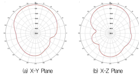
그림 15. 방사패턴 (선형편파, 수평방향) Fig 15. Radiation Pattern (LP, Horizontal)
