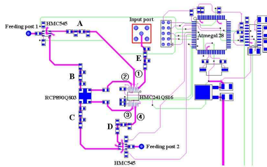
그림 9. PADS를 이용하여 설계된 회로도면 Fig 9. Designed schematic by using the PADS
