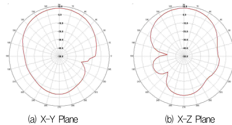
그림 16. 방사패턴 (선형편파, 수직방향) Fig 16. Radiation Pattern (LP, Vertical)
