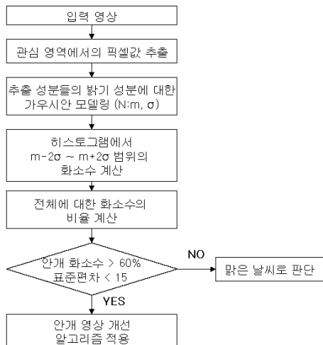
그림 3. 안개 영상 판단 알고리즘의 흐름도 Fig. 3. Flowchart for fog judgment algorithm
