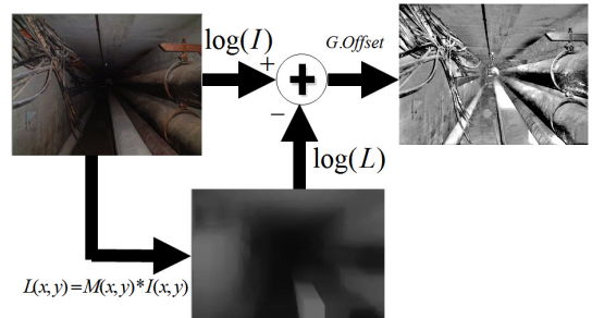
그림 7. 미디언 필터 기반의 Retinex 알고리즘 과정 Fig. 7. Median filter based Retinex algorithm
