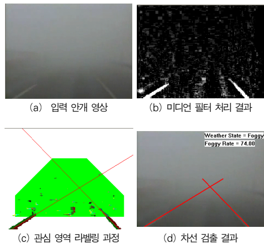
그림 10. 안개 영상의 차선 검출 결과 Fig. 10. Lane detection for foggy image
