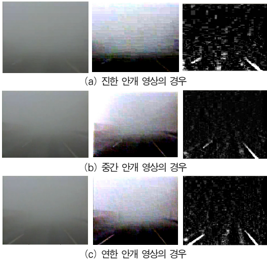
그림 11. 3가지 안개 상태에 대해 가우시안 필터와 미디어 필터 기반의 Retinex 알고리즘 적용 결과 비교 Fig 11. Comparison for foggy image between Gaussian filter and Median filter based Retinex
