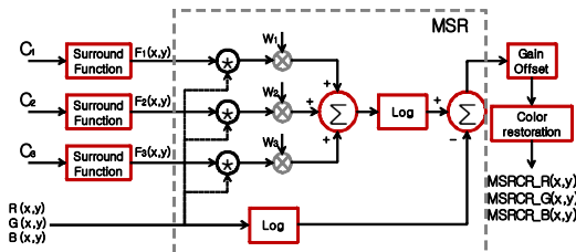
그림 5. MSR 알고리즘의 블록 다이어그램 Fig. 5. Block diagram for MSR of Retinex method
