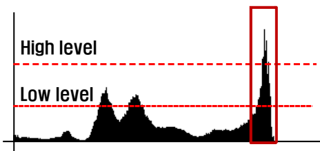
그림 9. 이중 임계치를 이용한 이진화 과정 Fig. 9. Binarization using Multi threshold
