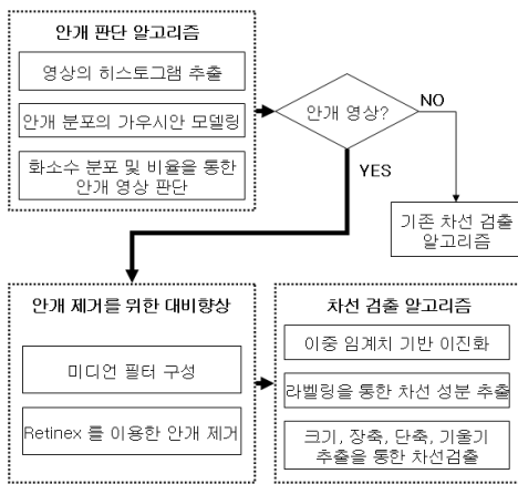
그림 1. 제안된 차선 검출의 전반적 흐름도 Fig. 1. Overall Flowchart for Proposed Lane Detection.
