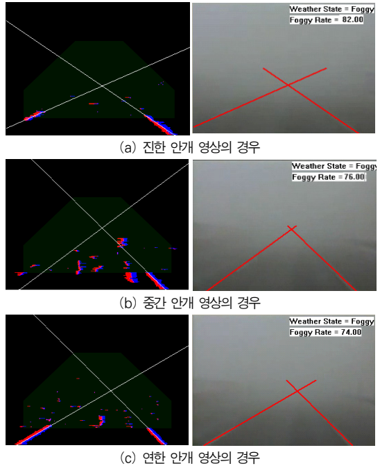
그림 12. 그림 11의 3가지 안개 상태에 대해 제안된 알고리즘을 적용하여 차선 성분을 검출한 결과 Fig 12. The result of lane detection for three kind of foggy condition (as shown Fig 11) using Median filter based Retinex algorithm
