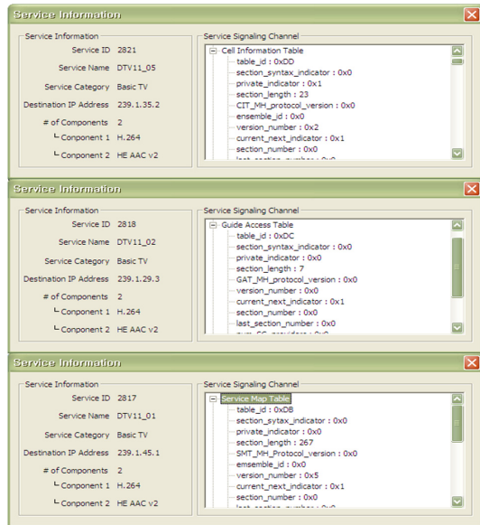
그림 9 (b). Monitoring System 서브다이얼로그화면 Fig. 9 (b). Screen of Monitoring System Sub Dialog
