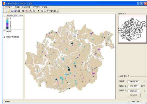
그림 7. 티부서치 변형 모델에 의해 선정된 최적 시업대상지 Fig. 7. Harvest units resulted from the revised Tabu Search model
