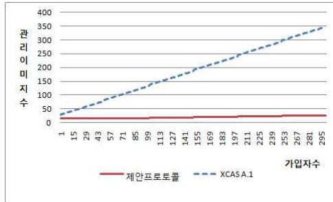
그림 10. 제안프로토콜과 XCAS A.1의 XCAS Server에서 관리하는 이미지 수 비교 Fig. 10. Image count Comparison for managing Proposed Protocol and XCAS A.1
