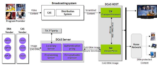
그림 1. DCAS 구성도 Fig. 1. DCAS configuration
