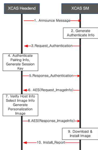
그림 6. 업데이트 다운로드 프로토콜 Fig. 6. Update download protocol
