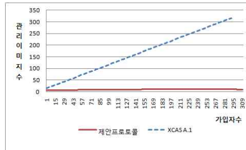
그림 8. 제안프로토콜과 XCAS A.1의 XCAS Server에서 관리하는 이미지 수 비교
