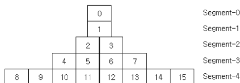
그림1. 피라미드 세그먼트화 Fig. 1. Pyramid Segmentation
