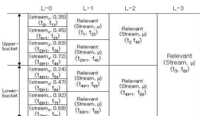
그림3. 멀티-레벨 스트림 구조 Fig. 3. Multi-level Stream Structure
