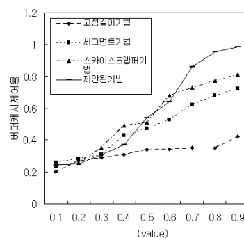
그림5. 버퍼캐시 제어율
