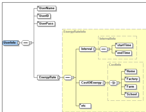
그림 3. 사용자 모델링 Fig. 3. User Modeling
