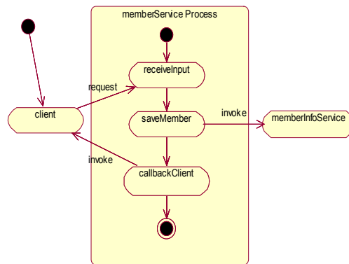
그림 6. memberService 액티비티 다이어그램 Fig. 6. memberService Activity Diagrams
