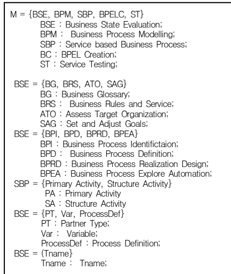
그림 1. 모델 구성요소 Fig. 1 Model Elements
