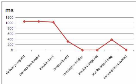
그림 10. 스트레스 테스트 추함 Fig. 10. Stress Test Result
