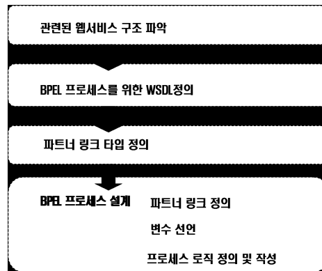
그림 3. BPEL 설계 Fig. 3 Design of BPEL
