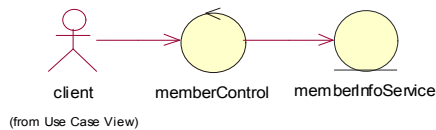
그림 5. memberService의 클래스 다이어그램(클래스 뷰) Fig. 5. memberService Class Diagrams (Class View)
