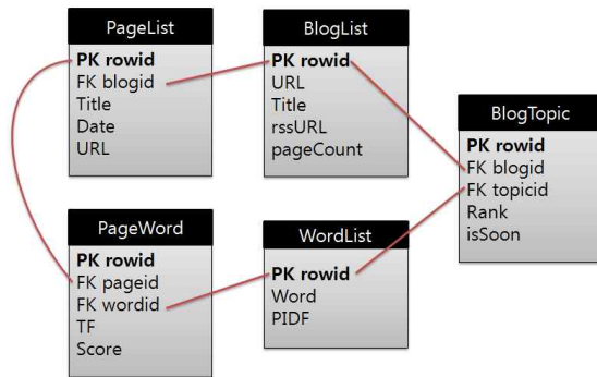
그림 2. 데이터베이스 스키마 Fig. 2. Database Scheme.
