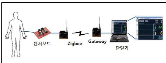
그림 4. 무선 센서네트워크 구성 Fig. 4. Structure of WSN
