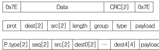
그림 5. 패킷 형태 Fig. 5. Packet Format
