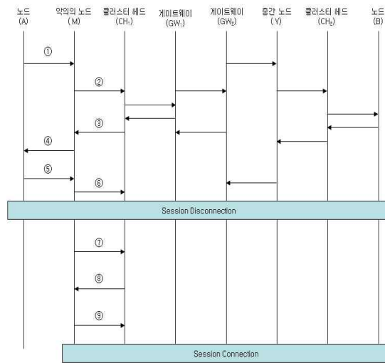
그림 3. 클러스터에서 재생 공격 Fig 3. Replay Attack in cluster
