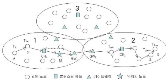
그림 1. 본 논문의 네트워크 구조 Fig 1. Network Environments
