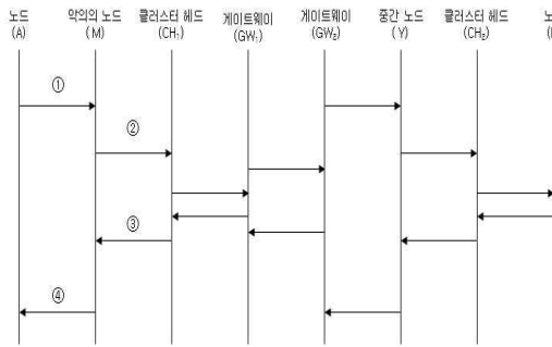
그림 2. 클러스터에서 중간자 공격 Fig 2. Man-in-the-middle Attack in cluster
