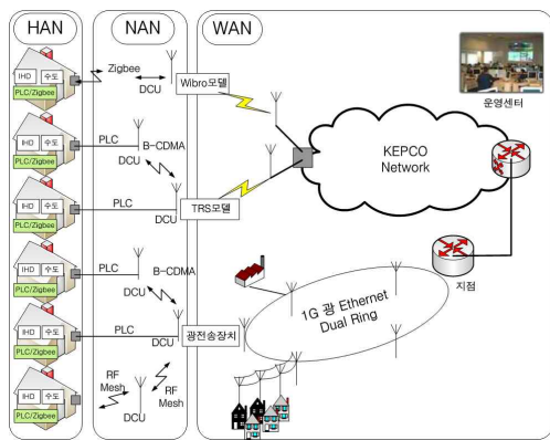
그림 1. 통신망 및 운영센터 구성도 Fig 1. Architecture of communications network and Operation Center architecture.
