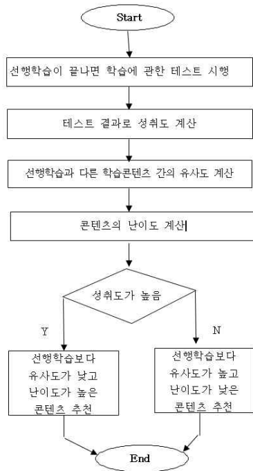
그림 1. 콘텐츠 추천 프로세스 Fig. 1. Content recommendation Process
