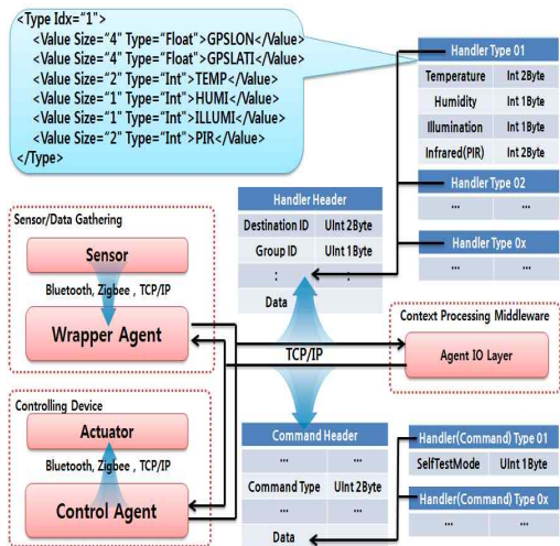
그림 3. 에이전트와 미들웨어의 통신 방법 Fig. 3. Communication method between agents and middleware
