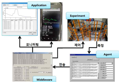
그림 9. 철로 감시 시스템의 실험 Fig. 9. An experiment of railroad monitoring system
