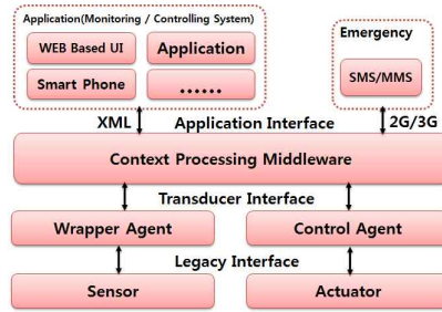
그림 1. 상황 인식 시스템의 구성도 Fig. 1. Architecture of context-aware system
