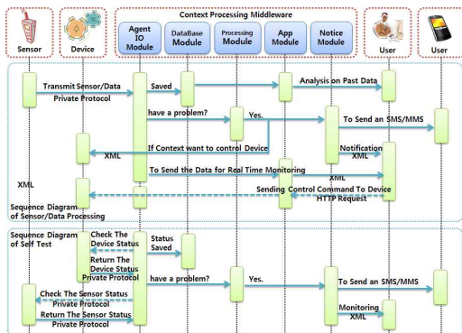
그림 6. 미들웨어의 상황정보 처리 Fig. 6. Context Information processing of middleware
