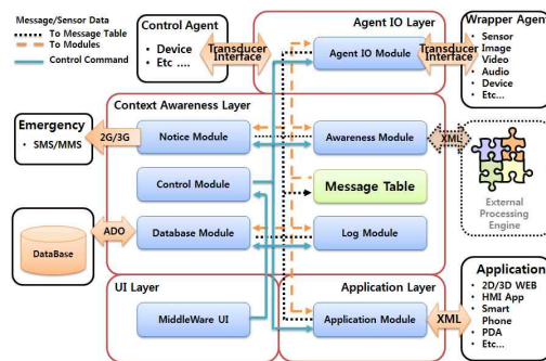
그림 2. 상황 인식 미들웨어의 구조 Fig. 2. Architecture of context-aware middleware
