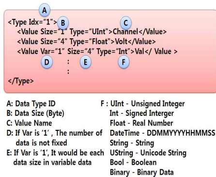
그림 4. 상황 정보 정의를 위한 XML의 구조 Fig. 4. XML structure for definition of context information
