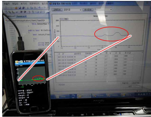
그림 10. 측정된 값의 스마트폰과 PC프로그램 비교 Fig. 10. Result view comparison between Smart-phone and PC application
