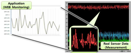
그림 8. 측정된 센서와 모니터링 값의 비교 Fig. 8. Comparison between real sensor data and web monitoring data
