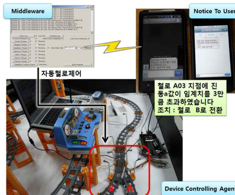
그림 11. 철로 감시 시스템의 응급상황 실험 Fig. 11. An experiment of emergency situation of railroad monitoring system
