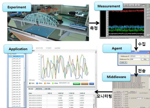
그림 7. 교량 건전성 감시 시스템의 실험 Fig. 7. An experiment of bridge health monitoring system
