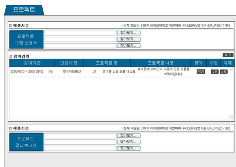
그림 8. 프로젝트 관리 기능 Fig. 8. Project Management Function.
