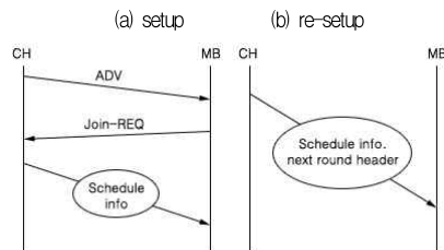
그림 3. 제안방식의 셋업과 재셋업 과정 Fig. 3. Setup and re-setup process of the proposed protocol
