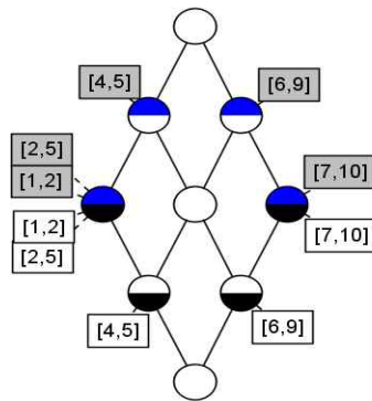
그림 3. 개념격자 B(TK(m_3, 5)) Fig. 3. Concept Lattice B(TK(m_3, 5))
