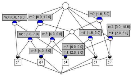
그림 4. 표8로부터 추출된 개념격자 Fig. 4. Concept Lattice extracted from Table 8
