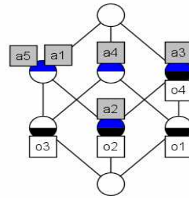
그림 1. 표1의 데이터테이블에 대한 개념격자 Fig. 1. Concept Lattice for Data Table 1
