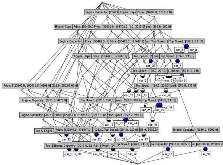
그림 10. 표9의 임계값 집합을 37가지 속성(Price, Engine Capacity, Top Speed)에 적용하여 생성된 분류체계
