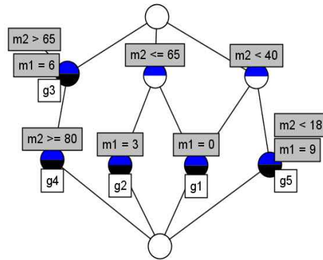
그림 2. 표5의 개념격자 Fig.2. Concept Lattice of Table 5
