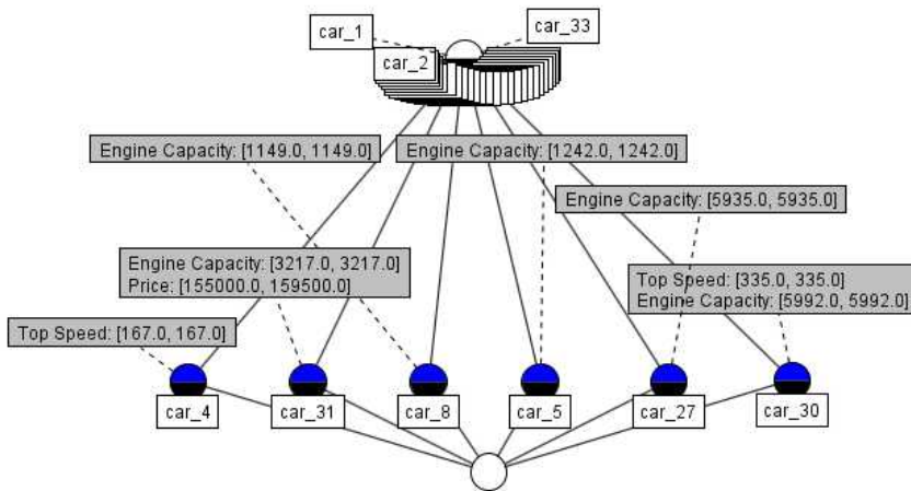
그림 9. 표9의 임계값 집합을 3가지 속성(Price, Engine Capacity, Top Speed)에 적용하여 생성된 분류체계 Fig. 9. Classification Hierarchy generated by applying the threshold value set I of Table 9 on the three attributes(Price, Engine Capacity, Top Speed)
