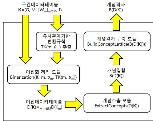
그림 6. 지원도구(iFCA)의 구성도 Fig. 6. Architecture of Supporting Tool(iFCA)
