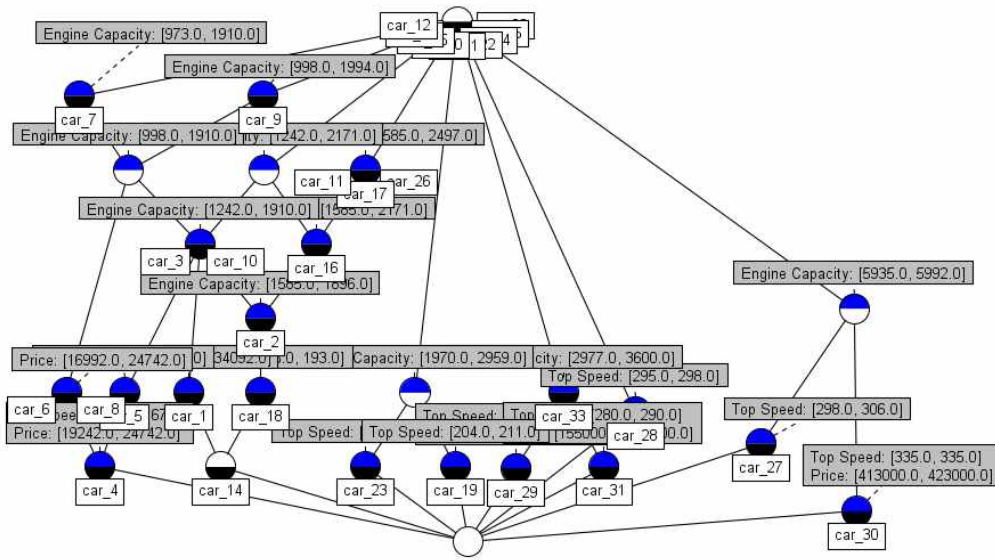
그림 11. 표9의 임계값 집합III을3가지 속성(Price, Engine Capacity, Top Speed)에 적용하여 생성된 분류체계 Fig. 11. Classification Hierarchy generated by applying the threshold value set III of Table 9 on the three attributes(Price, Engine Capacity, Top Speed)
