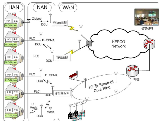
그림 1. 통신망 및 운영센터 구성도 Fig 1. Architecture of communications network and Operation Center architecture.
