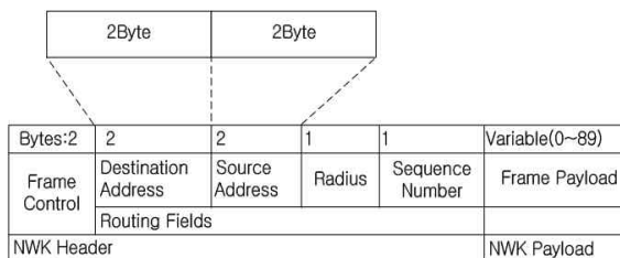
그림4. 네트워크 계층의 프레임 형식 Fig.4. The network layer frame format
