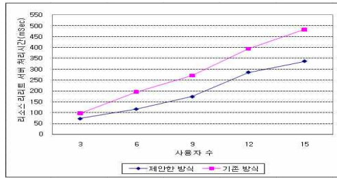
그림 9 SIP NOTIFY 메시지 처리 시간 Fig. 9 SIP NOTIFY Message Processing Time
