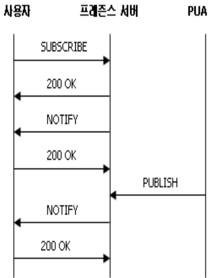
그림 2 SIP 통지 메시지 Fig. 2 SIP Notification Message
