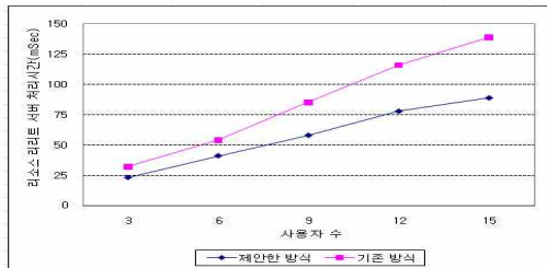
그림 10 rsc-match-entity 효과 비교 Fig. 10 Comparison of rsc-match-entity Effect
