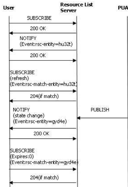
그림 6 통지 메시지 억제 동작 Fig. 6 Suppress operation of Notification Message
