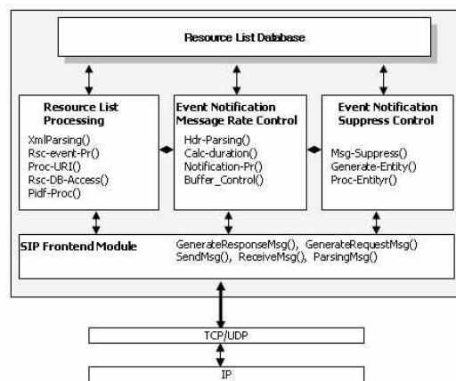
그림 7 구현된 리소스 리스트 서버의 기능 블록 Fig. 7 Function Block of Implemented Resource Lists Server
