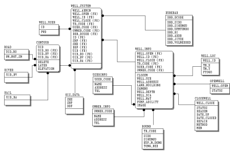
그림 7. 데이터베이스 개체-관계 다이어그램 Fig. 7. Entity-Relationship Diagram for Database
