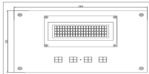
그림 4. 제어보드 설계도 Fig. 4. Blueprint of Control Board
